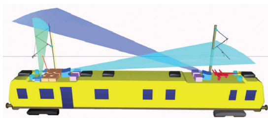
Prinzipieller Messsystem-Aufbau
