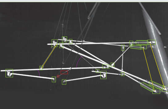
Inspektionsergebnis Quertragwerk
